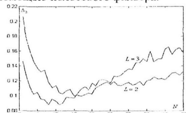
Рис.7. Погрешности сплайнового фильтра
