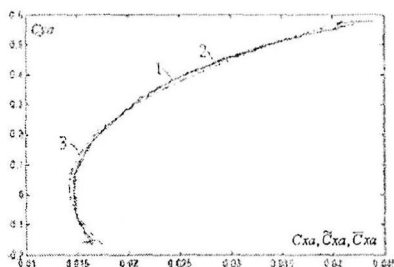
Рис.2. Исходная (1), сплайновая аппроксимация (2) и параболическая аппроксимация (3) поляры c_{ju}(i) = P_0(c_{xa}(i))
