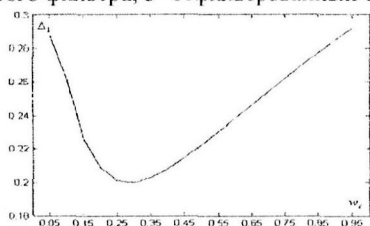
Рис.6. Погрешности полосового фильтра
