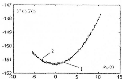
Рис. 4. Аппроксимационная сплайновая фильтрация зависимости подъёмной силы
