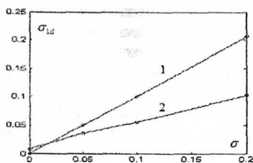
Рис.10. Сравнительные оценки СКЗ погрешностей алгоритмов преобразования частоты дискретизации
