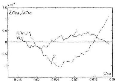
Рис.3. Функции погрешностей цифровой фильтрации, сплайновая аппроксимация (1), параболическая аппроксимация (2)
