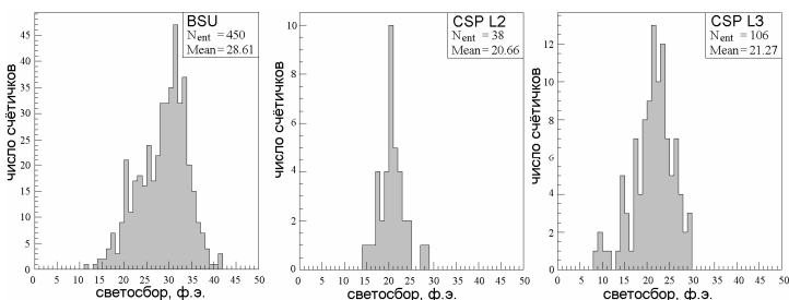
Рис. 9. Светосбор с дальнего от ФЭУ конца для сцинтилляционных счётчиков BSU, CSP L2 и CSP L3 типов, изготовленных в ОИЯИ.
