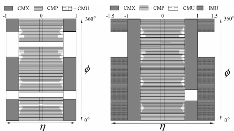
Рис. 11. Акцептанс мюонной системы CDF в Run I – слева и в Run II – справа.
