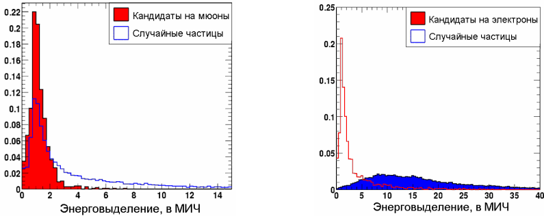
Рис. 16. Распределение по выделенной в преконверторе энергии (в единицах МИЧ) для кандидатов на мюоны от распадов W -бозонов и от случайных треков с поперечной энергией p_t более 8 \text{ ГэВ} (левый рисунок). То же для кандидатов на электроны от распадов W -бозонов и от случайных частиц с поперечной энергией p_t более 8 \text{ ГэВ} (правый рисунок).
