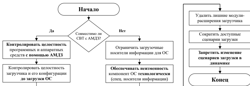
Рисунок 1 – Блок-схема алгоритма доверенной загрузки загрузчика и ОС
