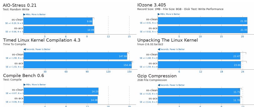
Рисунок 4 – Диаграммы сравнения результатов нагрузочных тестов в ОС Linux до и после внедрения средства разграничения доступа
