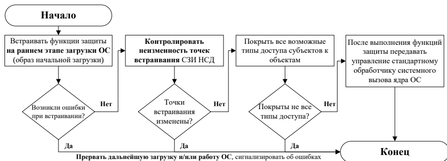
Рисунок 2 – Блок-схема алгоритма встраивания функций защиты от НСД на раннем этапе загрузки ОС
