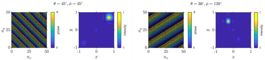
Рис. 2. Распределение фазы вдоль метаповерхности и распределение интенсивности в дальнем поле при различных значениях углов \theta и \phi
