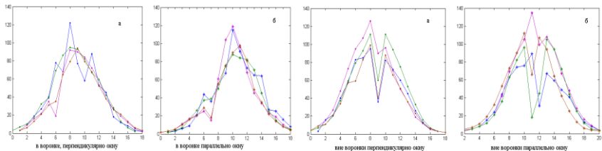
Рис. 2. Распределение интенсивности по поперечному сечению лазерного луча: первые два графика – лазер в «фантомном» поле в двух взаимноперпендикулярных направлениях, вторые два графика – лазер вне фантомного поля в тех же направлениях
