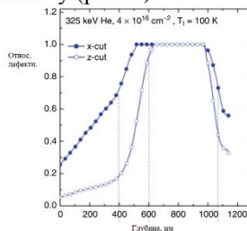
Рис. 2. Распределение дефектов структуры НЛ по глубине (отн.ед. 1.0 – аморфное состояние) [3]
