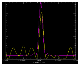
Рис. 3. Разделение ЛЧМ-сигнала на 2024 сегмента
