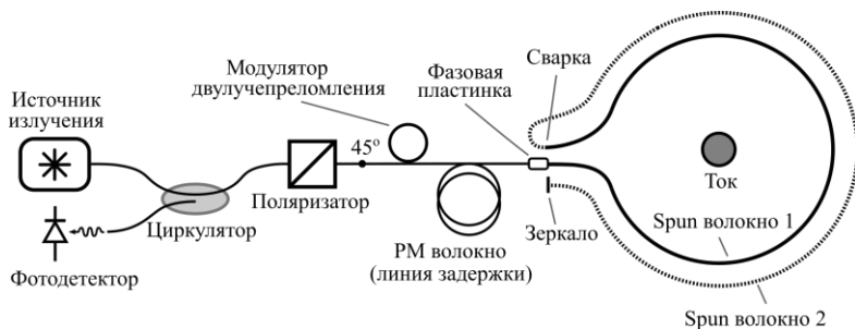
Рис. 1. Схема датчика
