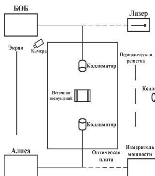
Рис. 1. Экспериментальная установка
