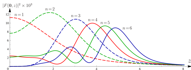
Рис. 1. Графики зависимости интенсивности |F(\mathbf{0}, z)|^2 от z при выборе параметра смещения 3^{2/3} a = a'_n и 1 \leq n \leq 6 , точка глобального максимума характеризует местоположение плоскости автофокусировки z_s , при n = 1 такой плоскости нет, для остальных n плоскость существует и величина z_s с ростом n монотонно растёт
