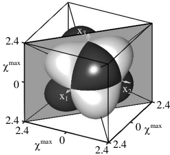
Рис. 1. Поверхность \chi^{\max}(\mathbf{K})
