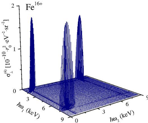
Рис. 1. Четырёхжды дифференциальное сечение расщепления фотона ионом \text{Fe}^{16+} для \perp -схемы эксперимента. Энергия падающего фотона \hbar\omega = 9 keV [1], \hbar\omega_{1,2} – энергии рассеянных фотонов, энергия порога ионизации 1s^2 -оболочки I_{1s} = 7.7 keV, естественная ширина распада 1s – вакансии \Gamma_{1s} = 1.046 eV [2]
