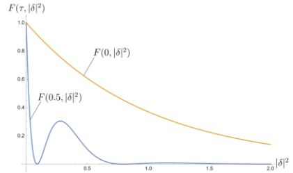
Рис. 2. Зависимость функции квантовой чувствительности от сдвига |\delta|^2 в случае, когда накачка моды a_2 неистощимая, в начальный момент времени мода a_1 находится в состоянии кота Шредингера с |\alpha_{10}|^2 = 5 и \arg(\alpha_{10}) = 0 . \tau = 0.5
