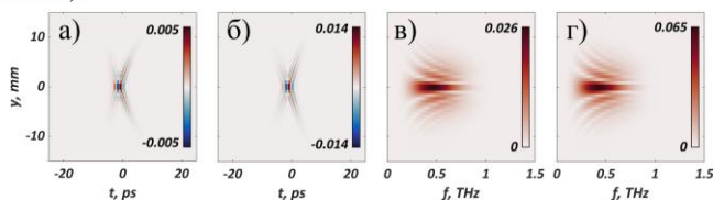
Рис. 1. Пример пространственно-временных (а, б) и пространственно-спектральных сечений поля (в-г), полученных в моделировании при сканировании поля диафрагмой (а, в) и системой «диафрагма-линза» (б, г)
