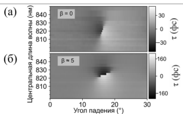
Рис. 2. \lambda - \theta зависимости задержки \tau лазерных импульсов для \beta = 0 (а) и \beta = 5 (б)
