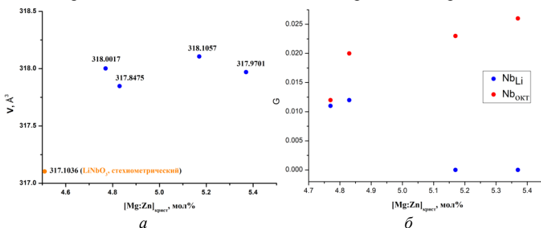
Рис. 1. Концентрационная зависимость объёма элементарной ячейки ( a ); концентрационная зависимость количества точечных дефектов ( \text{Nb}_{\text{Li}} , \text{Nb}_{\text{Okt}} ) ( b )
