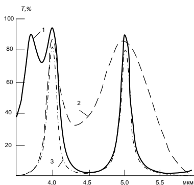
Рис. 2. Спектры пропускания: отсекающий фильтр (1), интерференционный фильтр (2), результирующий спектр (3)
