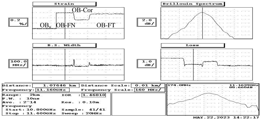
Рис. 2. Мультирефлектограмма для световода с G.654
