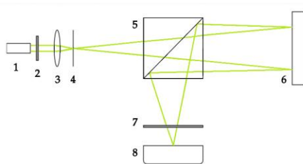
Рис. 1. Установка: 1 – лазер; 2 – ослабляющий фильтр; 3 – собирающая линза; 4 – апертура; 5 – светоделительный куб; 6 – модулятор; 7 – поляризатор, 8 – камера
