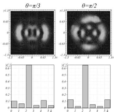
Рис. 2. Экспериментально полученная карта распределения поляризации векторного сЛГ пучка для (n, l) = (5, 1) и спектры ЭГ мод сЛГ пучка в \hat{x} поляризационных компонентах
