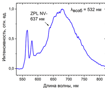
Рис. 2. Спектр фотолюминесценции на кончике микроструктуры
