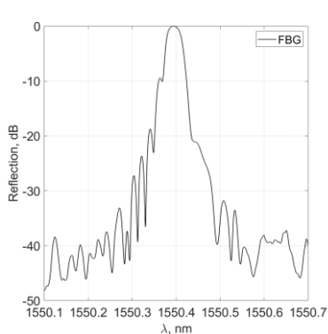
Рис. 2. Спектр волоконной брэгговской решётки
