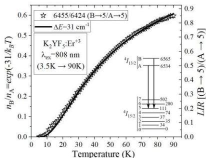
Рис. 1. LIR переходов ( B \rightarrow 5 ) и ( A \rightarrow 5 ) отношения населенностей n_B/n_A в бальцмановском распределении
