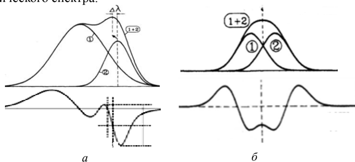
Рис. 1. Спектральные ситуации, складывающие при исследовании многокомпонентных образцов: наложение спектральных линий (а); перекрывающиеся близко расположенные спектральные линии (б)
