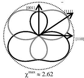
Рис. 2. Сечение поверхности \chi^{\max}(\mathbf{K})
