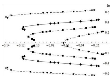
Рис. 2. Зависимость внешних поперечных волновых чисел вытекающих мод (трёх наименьших по модулю) на длине волны \lambda = 1.55 \mu\text{m} (1●), (2▼), (4◆) и одного на \lambda = 2 \mu\text{m} (3■) от значений n_2 = 1 (1), 1.36 (7), 1.453 (12)
