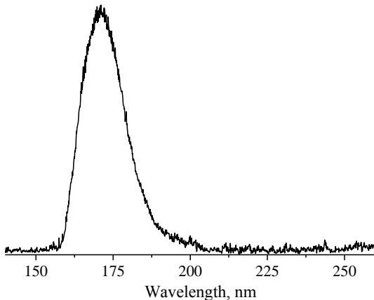
Рис. 1. Спектр излучения эксимерной лампы
