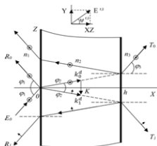
Рис. 1. Схема считывания ГР в слое (XZ – плоскость дифракции, R_0, R_1 – коэффициенты отражения, T_0, T_1 – коэффициенты пропускания, \varphi_1 (\varphi_2) – угол падения (преломления), \varphi_3 – угол преломления)
