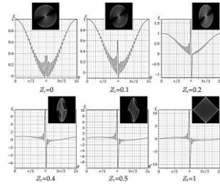
Рис. 2. Осцилляции ОУМ \xi_z(\theta) при вариации \theta -управляющего параметра аСЛГ пучка с n = 20 , \ell = 1 , \varepsilon = 1 на различных длинах пучка Z_1 , выноски: картины интенсивности для первого всплеска ОУМ
