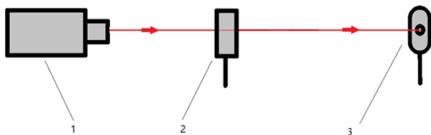
Рис. 1. Схема установки для измерения мощности излучения лазера: 1 – иттербиевый волоконный лазер ЛК-100-ЛП-ОМ-В; 2 – диафрагма со светофильтрами; 3 – измерительная головка ОРНН 3А КТ2017011-1-28
