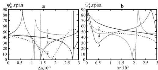
Рис. 2. Зависимость азимутов поляризации прошедшей дифрагированной волны нулевого порядка \psi_0^t (а) и первого порядка \psi_1^t (б) на ГР в слое от амплитуды изменения показателя преломления \Delta n при различных толщинах слоя h : 1 (1), 1.5 (2), 2 (3), 2.5 мм (4) (кристалл GaAs , n_1 = n_3 = 1 , n_2 = 3.18 , \lambda_0 = 1.15 мкм, \varphi_1 = 2^\circ , \psi_0 = 45^\circ )
