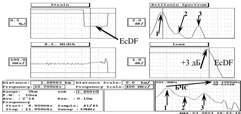
Рис. 2. Мультирефлектограмма для ЕсDF
