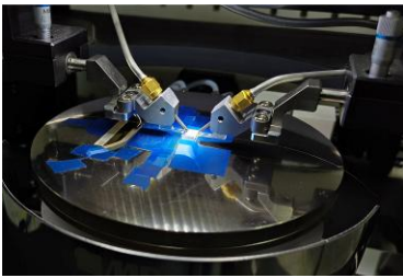
Рис. 1. Фазовый ТПНЛ модулятор, изготовленный в ФТИ им. А.Ф. Иоффе
