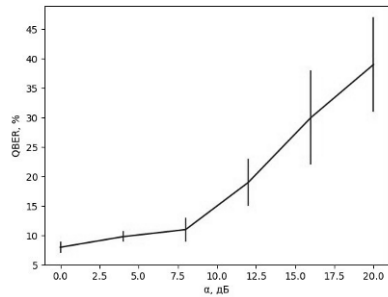
Рис. 2. Зависимость среднего QBER от затухания
