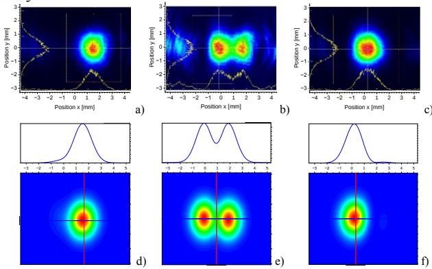
Рис. 1. Измеренные (a, b, c) и рассчитанные (d, e, f) профили интенсивностей отражённого пучка, прошедшего через фильтр LCP на расстоянии z = 25 см от дифракционной структуры: \theta_i = \theta_{\text{res}} = 33.53^\circ , \gamma = -4^\circ (a, d), \gamma = 0^\circ (b, e), \gamma = 4^\circ (c, f)
