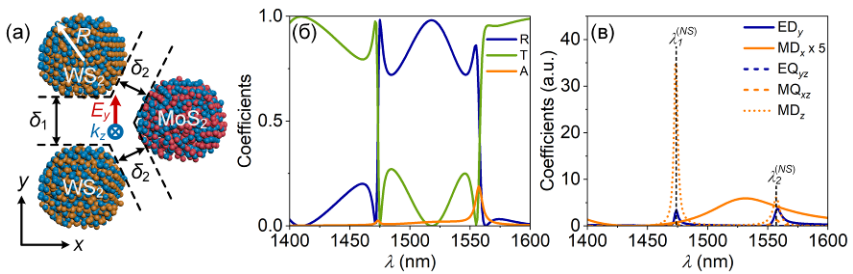
Рис. 1. Структура тримера из сферических MoS_2 и WS_2 наночастиц (а); спектры отражения, пропускания и поглощения (RTA) метаповерхности с периодами P_x = 1046 нм и P_y = 1094 нм, составленной из тримеров частиц с радиусами R = 200 нм и расстояниями между частицами \delta_1 = 50 нм, \delta_2 = 30 нм, облучаемой плоской волной с поляризацией E_y(k_z) (б); мультипольная декомпозиция отдельного тримера из метаповерхности, приведены, как вклады основных компонент в RTA, так и вклад MD_z , для бианизотропной компоненты (в)
