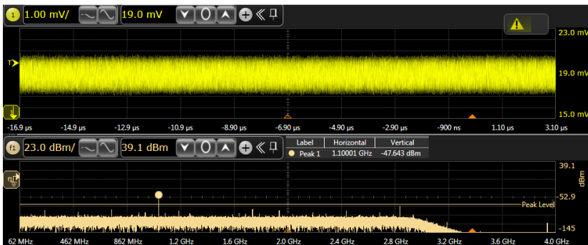
Рис. 2. Осциллограмма (сверху) и спектр (снизу) конвертированного сигнала, полученного переносом тестового сигнала с частотой 5.1 ГГц с помощью сканирующего сигнала с частотой 4 ГГц
