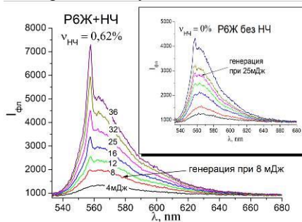
Рис. 1. Спектры излучения красителя при разных энергиях возбуждения
