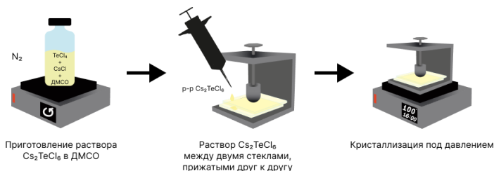
Рис. 1. Схематическая иллюстрация метода получения микрокристаллов перовскита
