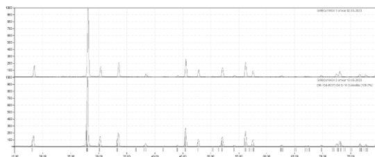
Рис. 1. Рентгеновские дифракционные спектры твёрдого раствора \text{Sr}_{1-x}\text{Ca}_x\text{WO}_4 ( x = 0,01 мол.%)
