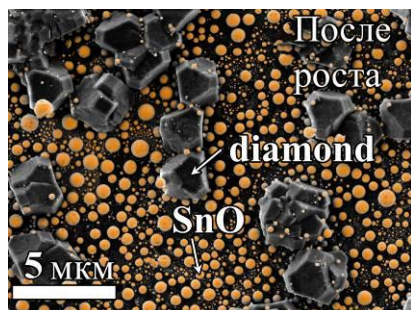
Рис. 1. РЭМ-изображение выращенных алмазных микрочастиц на подложках AlN
