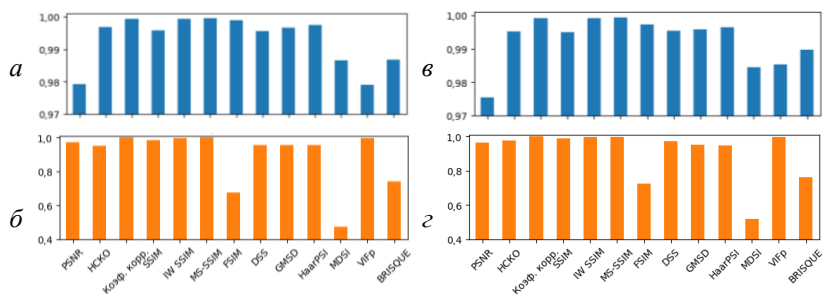
Рис. 1. Коэффициенты корреляции Пирсона (а, в) и Спирмена (б, г) для восстановленных изображений с голограмм с добавленным шумами: «соль и перец» (а, б) и гауссовым (в, г)
