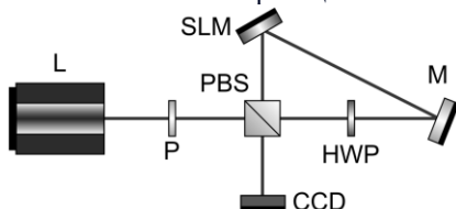
Рис. 1. Схема установки: L – полупроводниковый лазер 650 нм, P – поляризатор, PBS – поляризационный светоделитель, SLM – пространственный модулятор света, HWP – полуволновая пластинка, M – зеркало, CCD – камера с ПЗС-матрицей
