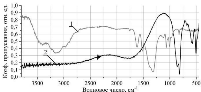
Рис. 1. ИК-спектры пропускания плёнок \text{BiFeO}_3 после предварительной сушки (1) и после термического отжига (2) в спектральном диапазоне 3800 - 450 \text{ см}^{-1}
