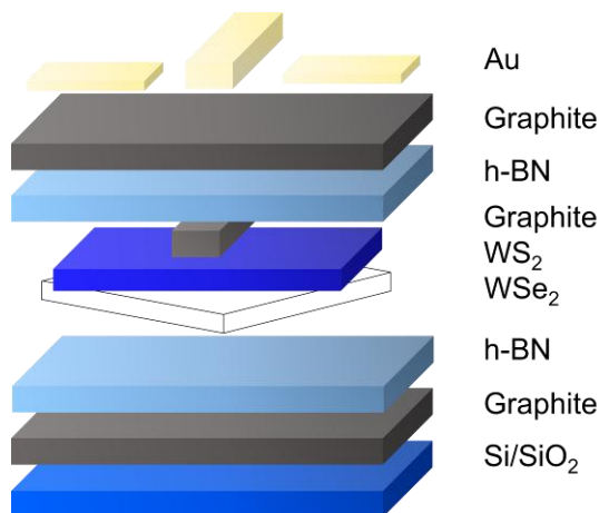
Рис. 1. Модель гетероструктуры на основе слоёв дихалькогенидов вольфрама со структурой Графит/hBN/ \text{WSe}_2 / \text{WS}_2 /Графит/hBN/Графит/Au
