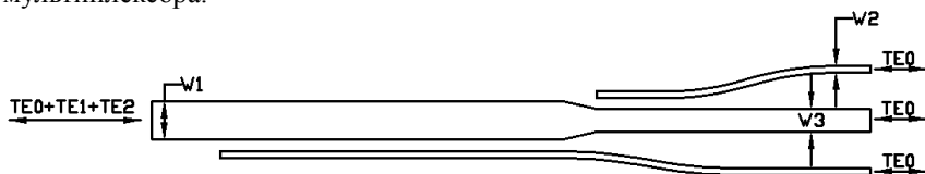
Рис. 1. Схематический вид волноводной структуры интегрально-оптического модового мультиплексора на основе направленных ответвителей
