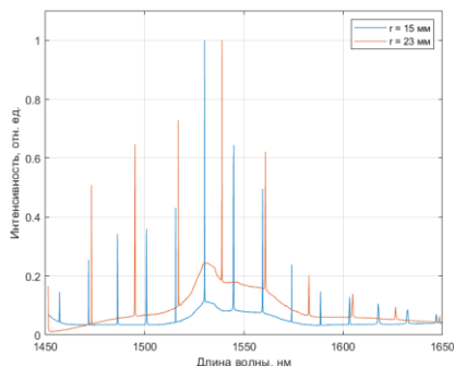
Рис. 2. Расчётные спектры люминесценции микрорезонатора из фосфатного стекла, легированного ионами эрбия
