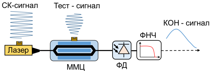
Рис. 1. Схема СВЧ-АОТ для переноса несущей частоты сигнала: ММЦ – модулятор Маха–Цендера, СК-сигнал – сканирующий сигнал (гетеродин), ФД – фотодиод, ФНЧ – фильтр нижних частот, КОН-сигнал – конвертированный сигнал
