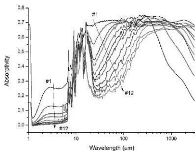
Рис. 1. Спектр поглощения Si пластин
