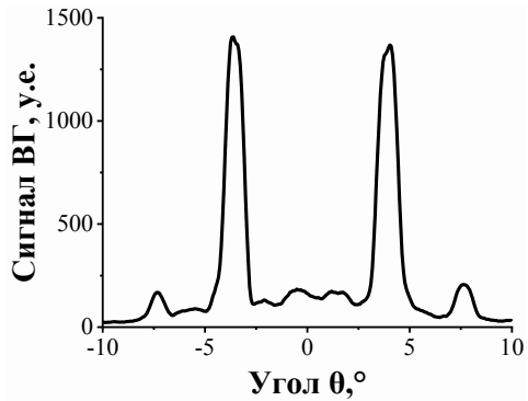
Рис. 2. Диаграмма направленности излучения ВГ для зарядовой структуры с шириной полосы 4 мкм при поляризации фундаментальной волны E_{\square}
