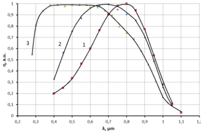
Рис. 1. Классические фотодиоды
