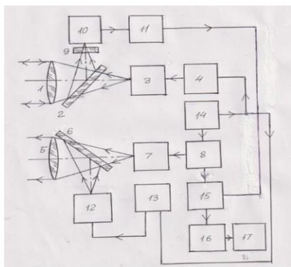
Рис. 1. Блок-схема ИЛО
