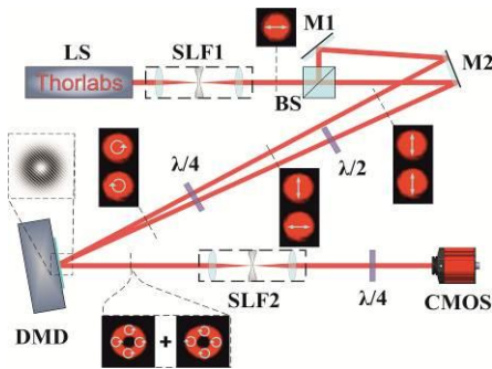
Рис. 1. Экспериментальная установка
