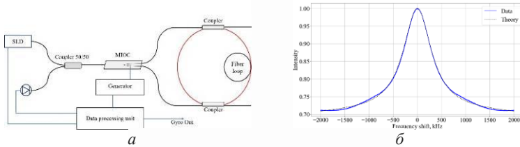
Рис. 1. Схема резонаторно-интерферометрического волоконно-оптического гироскопа (а); сравнение экспериментальной и теоретической зависимости изменения интенсивности РВОГ от частоты смещения (б)
