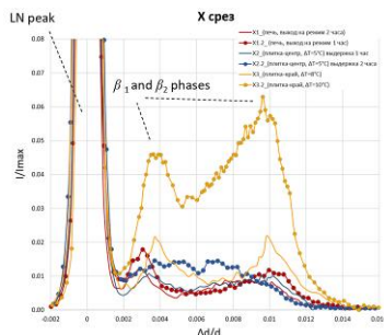
Рис. 2. Результат рентгеноструктурного анализа кристалла X-среза
