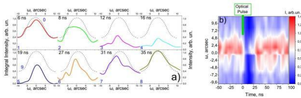
Рис. 2. Динамика изменения КДО при воздействии на ниобат лития, легированного железом, интенсивного наносекундного лазерного импульса (а, б)
