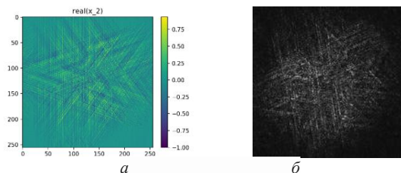
Рис. 2. Реальная часть фильтра с заданной формой в виде звезды (а) и распределение в первом порядке дифракции (б) соответствующего голографического фильтра, реализованного с помощью микрозеркального ПВМС
