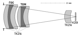
Рис. 1. Оптическая схема объектива
