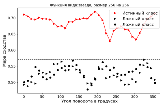
Рис. 3. Зависимость меры сходства полученной взаимокорреляционной функции и использованной при синтезе сглаживающей функции от угла поворота объекта на входном изображении
