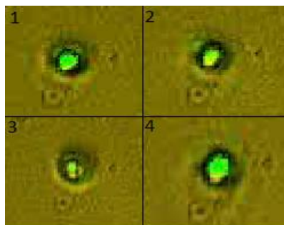
Рис. 2. Колебания частицы около положения равновесия в методе равновесного распределения
