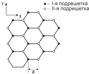
Рис. 1. Гексагональная двухподрешёточная двумерная решётка
