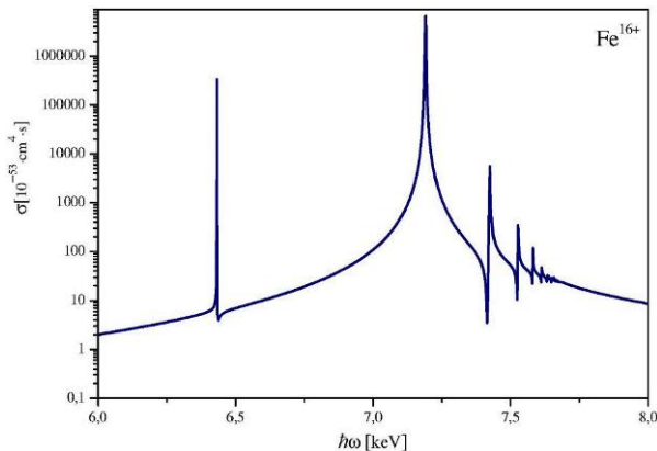
Рис. 2. Обобщённое сечение двухфотонной ионизации К-оболочки \text{Fe}^{16+}
