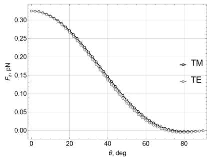
Рис. 4. Сравнение силы F_z , действующей на частицу с обычным рассеянием, при ТМ- и ТЕ-поляризациях
