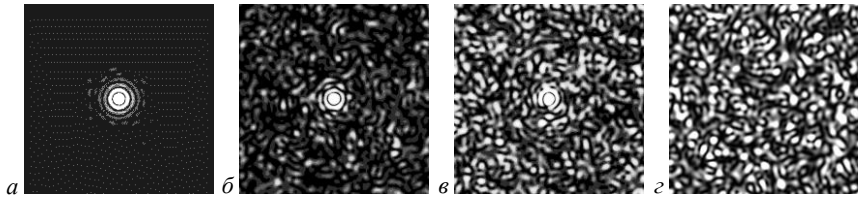
Рис. 1. Смоделированные спекл-картины волнового поля в поперечном сечении для круглой апертуры; интервал случайных начальных фаз \Delta\varphi и яркость спекл-картины: 0,4\pi , 95 % (а); 1,2\pi , 95 % (б); 1,4\pi , 95 % (в); 2\pi , 30 % (г); \lambda_0 = 0,55 мкм, числовая апертура NA_i = 0,5 ; размер фрагментов спекл-картин 20 \times 20 мкм
