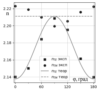
Рис. 2. Результат измерения n_o и n_e(\varphi) ТНЛ
