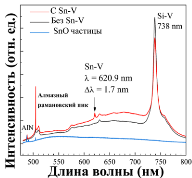
Рис. 2. Спектры фотолуминесценции при комнатной температуре выращенных: алмазных микрокристаллов с центрами Sn - V (красная кривая); алмазных микрокристаллов без центров Sn - V (чёрная кривая) и частиц SnO (синяя кривая)
