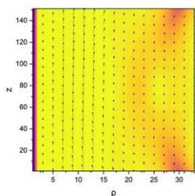
Рис. 1. Векторы ОУМ и распределение поляризационного параметра для правого вихря первого порядка
