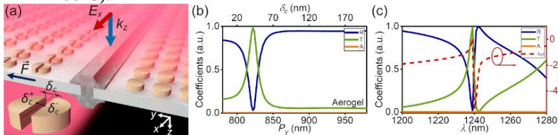
Рис. 1. Модель растяжимой метаповерхности из Si дисков с разрезом (a); зависимости коэффициентов отражения (R), пропускания (T) и поглощения (A) света метаповерхностью на подложке из аэрогеля от периода P_y . (b); спектральные зависимости коэффициентов R, T и A и набег фаз \Delta\varphi для метаповерхности при \delta_c = 40 нм, параметры метаповерхности: P_x = 780 нм, высота и диаметр целого Si диска 460 и 613 нм соответственно (c)
