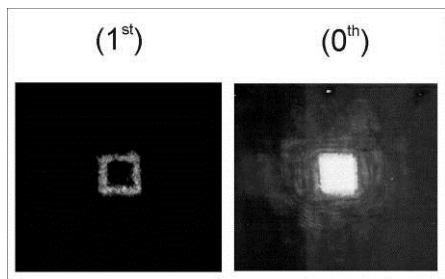
Рис. 1. Фотографии изображений после фурие-обработки, наблюдаемых на экране в первом ( 1^{\text{st}} ) и нулевом ( 0^{\text{th}} ) дифракционных порядках на частоте звука 9.95 МГц
