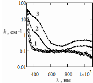
Рис. 1. Спектральные зависимости показателя поглощения в кристалле ниобата лития: 1 – чистый образец, 2 и 3 – легированные медью при T_1 = 600 °С и T_2 = 700 °С
