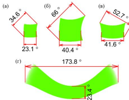
Рис. 1. Векторные схемы дифракции для различных схем ВГП: Hololens 1, n = 1,5 (а); Hololens 1, n = 1,8 (б); Hololens 2, n = 1,5 (в); схема с однокоординатной мультипликацией выходного зрачка, n = 1,5 (г)
