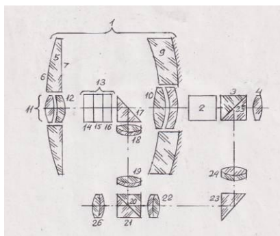
Рис. 1. Блок-схема ПНВ
