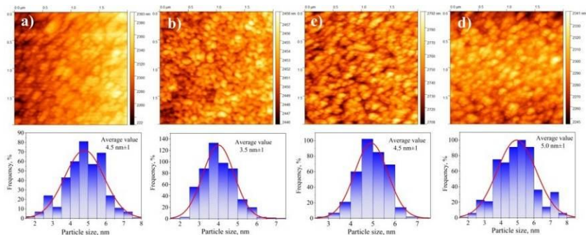
Рис. 1. АСМ-изображение поверхности и средний размер частиц плёнок NiO_x , отожжённых при 300 °С в воздухе (а), N_2 (б), O_2 (с), в вакууме (д)
