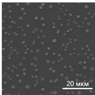
Рис. 1. СЭМ-изображение полученных кристаллов \text{CsGeI}_3
