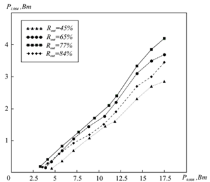
Рис. 2. Зависимости средней мощности излучения от поглощённой мощности накачки
