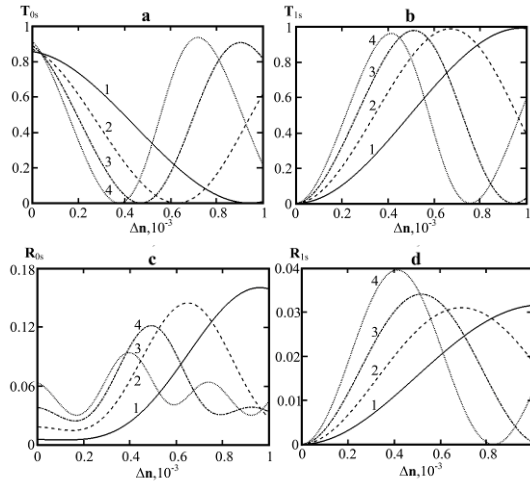
Рис. 1. Зависимости коэффициентов пропускания ( T_{0s} , T_{1s} ) и отражения ( R_{0s} , R_{1s} ) дифрагированной на голографической решётке световой волны в плоскопараллельном слое от фотоиндуцированного изменения показателя преломления \Delta n при различных толщинах слоя h : 1 (1), 1,5 (2), 2 (3), 2,5 мм (4) (реоксан, показатель преломления слоя – n_2 = 1,49 , показатель преломления покрытия и подложки – n_1 = n_3 = 1 , \lambda_0 = 0,6328 мкм, угол падения – \phi_1 = 2^\circ , азимут поляризации падающего света – \psi_0 = 45^\circ )
