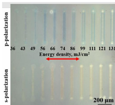
Рис. 2. Фотография дихроичных структур на ZnO:Ag плёнке
