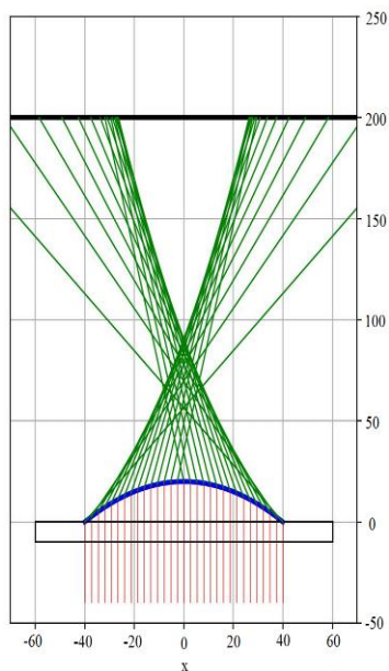
Рис. 2. Трассировка лучей через каплю со сферической поверхностью
