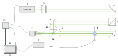
Рис. 1. Схема цифрового голографического комплекса для исследования апокамической плазмы в импульсном режиме генерации
