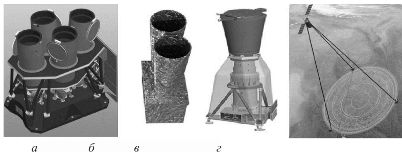
Рис. 1. Оптические конструкции объективов: Meteosat-12 (а); FY-4 (б); GOES (в); складной космический телескоп с мембранной оптикой (г)
