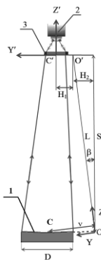
Рис. 1. Схема контроля внеосевой поверхности детали с ДОЭ
