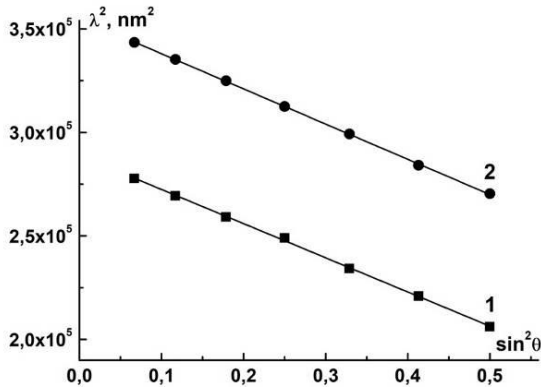
Рис. 1. Угловая дисперсия брэгговского резонанса первого порядка для исходной матрицы опала (кривая 1) и нанокompозита «сегнетоэлектрик / опал» (кривая 2)
