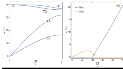
Рис. 1. Дисперсия продольной акустической (LA), поперечной акустической (TA), продольной оптической (LO) и поперечной оптической (TO) фононных веток решётки алмаза вдоль направления симметрии \Gamma - L , параметры (Н/м) [2]: a = 15.7 \times 10^4 ; b = 4.4 \times 10^4 ; l = -2.06 \times 10^4 ; \mu = 2.26 \times 10^4 ; \nu = 2.70 \times 10^4 ; \delta = 1.03 \times 10^4 (а); действительная и мнимая части квадратного корня первого собственного значения динамической матрицы при \mu = 0.16 \times 10^4 (б)
