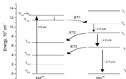
Рис. 2. Энергетические уровни \text{Nd}^{3+} и \text{Ho}^{3+}
