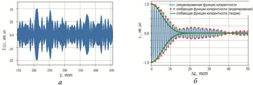
Рис. 1. Колебания немонохроматического волнового поля (а) и степень когерентности (б) при ширине спектра 100 нм и \lambda_0 = 920 нм
