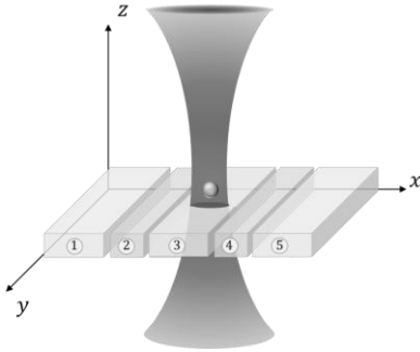
Рис. 1. Схема гибридной ловушки
