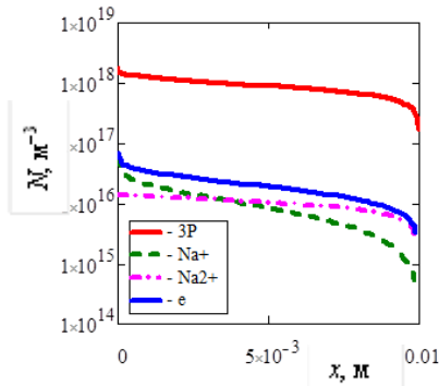
Рис. 1. Пространственные профили концентрации резонансных (3р) уровней натрия, ионов \text{Na}^+ и \text{Na}_2^+ и электронов
