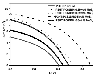
Рис. 1. Вольт-амперные характеристики устройств FTO/ZnO: P3HT: PC61BM: \text{MoS}_2 /PEDOT:PSS/Ag
