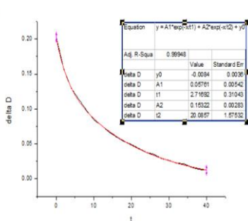
Рис. 1. Кинетическая кривая релаксации оптической плотности
