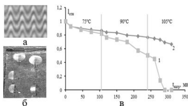
Рис. 1. Форма фоторельефа, наблюдаемого через интерференционный микроскоп (а); вид решёток при естественном освещении после термообработки (б) и кривые деградации относительной высоты рельефа (в)
