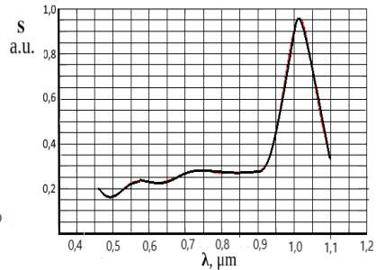
Рис. 4. Фотодиод с глубоким р-п переходом
