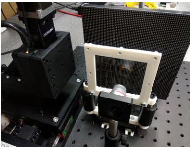
Рис. 1. Установка для оптической птихографии
