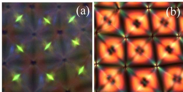
Рис. 1. Вид двумерного фотонного кристалла в отражённом (а) и проходящем (b) свете, поляризаторы скрещены, шаг спирали холестерика около 350 нм
