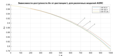
Рис. 2. Доступность терминалов АОЛС для дистанции 1 км
