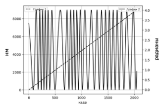
Рис. 1. График изменения интерференционного сигнала в центре изображения
