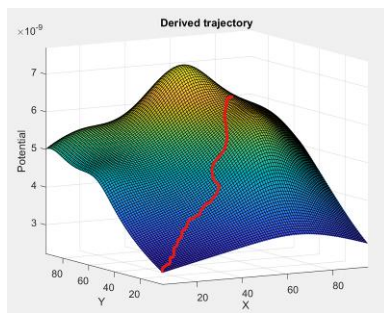
Рис. 2. Работа системы навигации по гравипотенциалу
