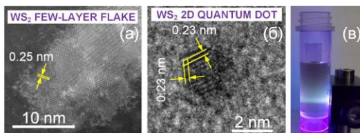
Рис. 1. ПЭМ-изображения: типичного \text{WS}_2 монослоя в NMP после 60 мин ультразвукового воздействия (а), \text{WS}_2 квантовые точки в ACN после 60 мин обработки лазерными фемтосекундными импульсами (б); фотолуминесценция раствора \text{WS}_2 в ACN после лазерной обработки (в)
