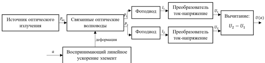
Рис. 1. Схема экспериментальной установки
