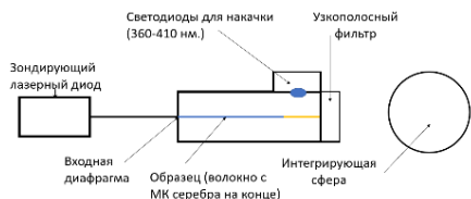
Рис. 1. Схема эксперимента по измерению усиления
