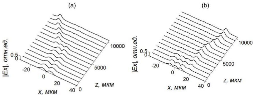
Рис. 2. Картина распространения мод TE_1 (a) и TE_2 (b) в модовом мультиплексоре
