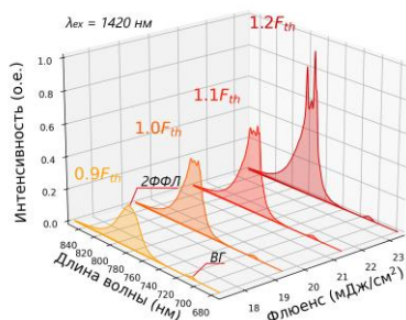
Рис. 2. Зависимость спектра двухфотонной фотолюминесценции от мощности вблизи порога лазерной генерации
