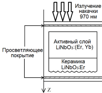
Рис. 1. Структурная картина, моделируемого устройства
