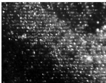
Рис. 1. Фрагмент микрофотографии поверхности X -грани образца \text{LiNbO}_3:\text{Cu} с агрегированными наночастицами \text{Al}_2\text{O}_3
